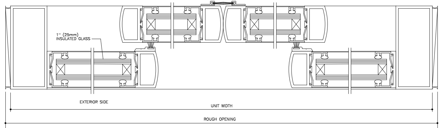
HORIZONTAL SECTION SCALE: FULL (2)
