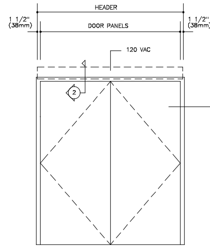
ELEVATION (4)
