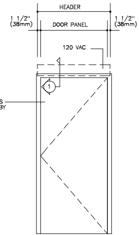
ELEVATION (6)
