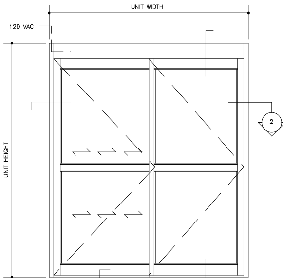
ELEVATION N.T.S.
