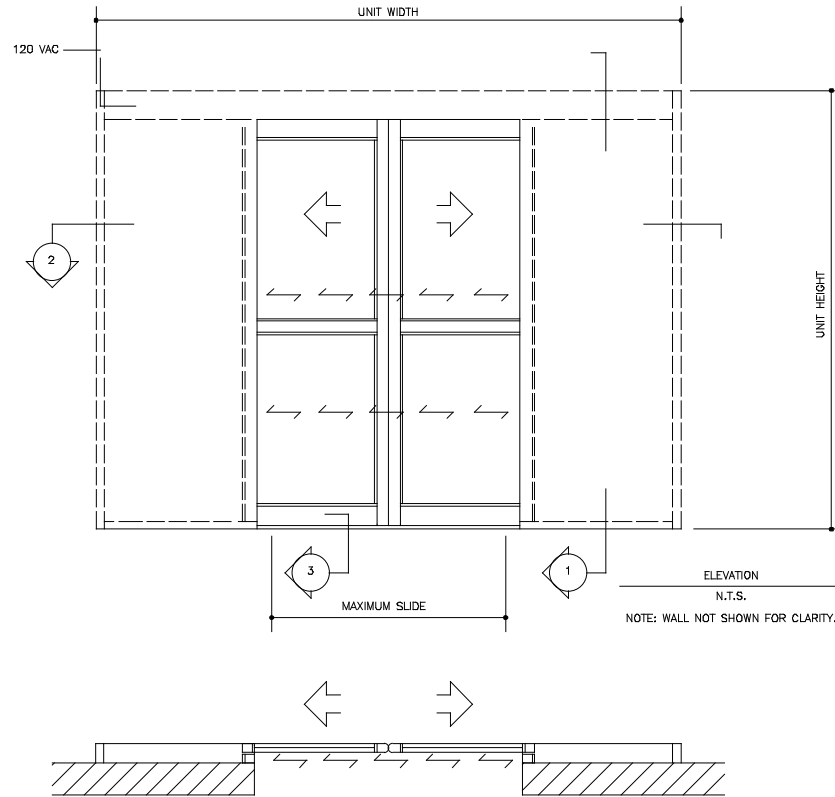
FLOOR PLAN N.T.S.
