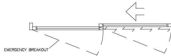
FLOOR PLAN N.T.S.
