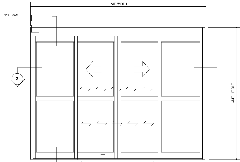
ELEVATION N.T.S.
