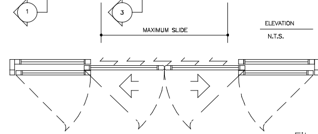
FLOOR PLAN N.T.S.
