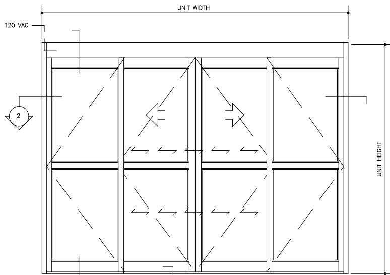
ELEVATION N.T.S.
