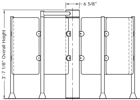
1 Elevation
